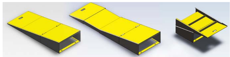
Collapsed 56" Long
